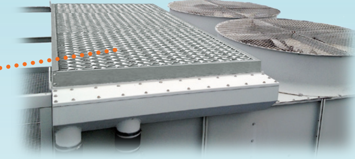
WST Louvers for Spray System Protection Griglie aspirazione aria WST a protezione del sistema di spruzzamento Grilles d'entrée d'air WST pour la protection du système de pulvérisation WST Lufteintrittsgitter zum Schutz des Sprühsystems
