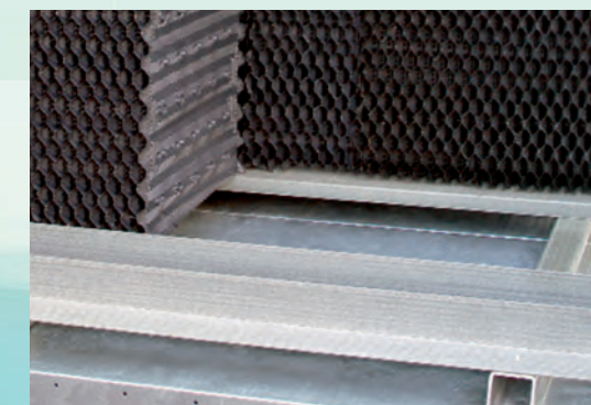
Possibile to Clean the Basin Possibilità di pulire il bacino Possibilité de nettoyer le bassin Reinigung des Beckens möglich
