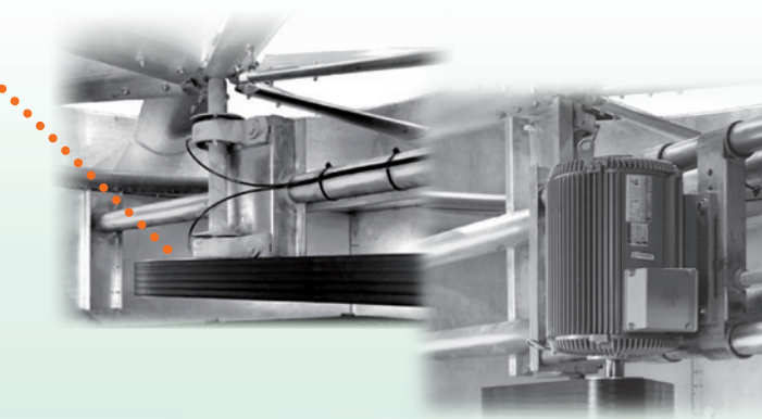
Fan Group Components Componenti del gruppo ventilante Composants du système d'entraînement Komponenten der Ventilatorsektion
